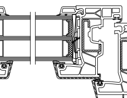
V8 = A030/76101(V309) - A036/76200(V315) - 76509
