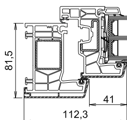
V1 = A030/76101(V309) - A036/76200(V315) - 76509
