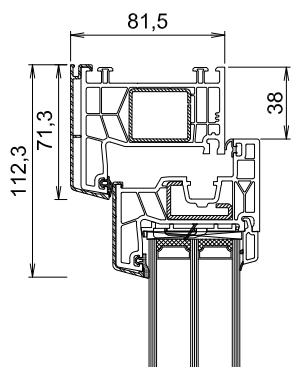
L1 = A030/76101(V309) - A036/76200(V315) - 76509
