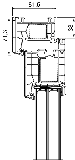
L20 = A030/76101(V309) - A038/76204(V326) - 76509
