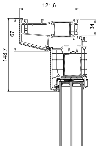
L20 = A576/76107(V381) - A038/76204(V326) - 76509
