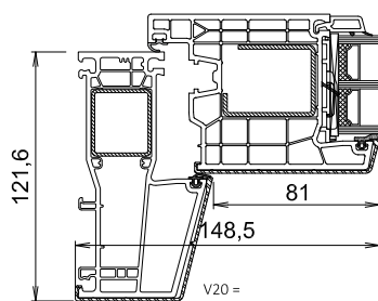
V20 = A576/76107(V381) - A038/76204(V326) - 76509
