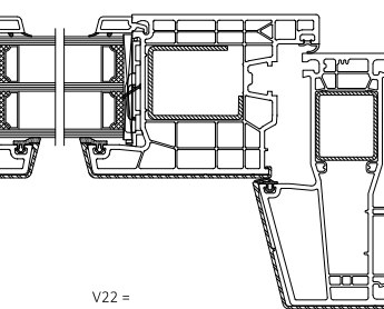
V22 = A576/76107(V381) - A038/76204(V326) - 76509
