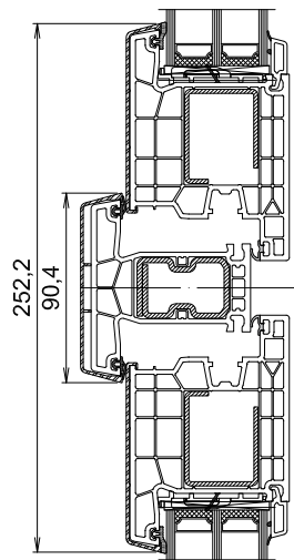
L4 = A038/76204(V326) - A046/76302(V319) - A038/76204(V326) - 76509
