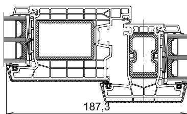
V3 = A046/76302(V319) - A040/76206(V260) - 76509
