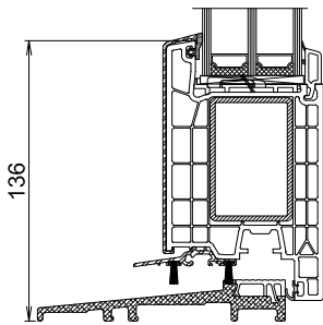
L22 = Z188/A061 - A040/76206(V260) - 76509
