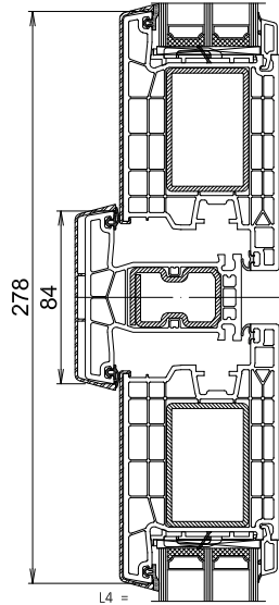
L4 = A040/76206(V260) - A046/76302(V319) - A040/76206(V260) - 76509
