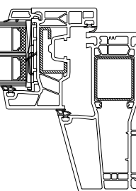
V8 = 76107(V381) - 76200(V315) - 76509
