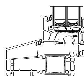
L8 = 76107(V381) - 76200(V315) - 76509
