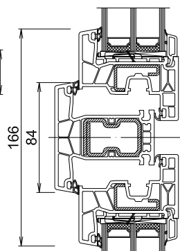
L4 = 76200(V315) - 76302(V319) - 76200(V315) - 76509
