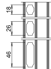
LS = ilagt sprosse 18 mm, 26 mm, 46 mm
