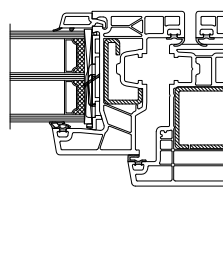
V9 = 76200(V315) - 76509 76402 (V310) 76200(V315) - 76509
