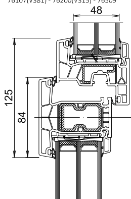
L2 = 76200(V315) - 76509 - 76302(V319) - 76509
