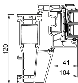
V1 = 76107(V381) - 76200(V315) - 76509
