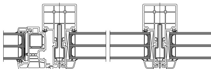
V3 = 76220(V556) - 76509 - 76318(V558) - 76505
