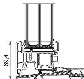
L22 = Z188/A575/A595 - 76220(V556) - 76509
