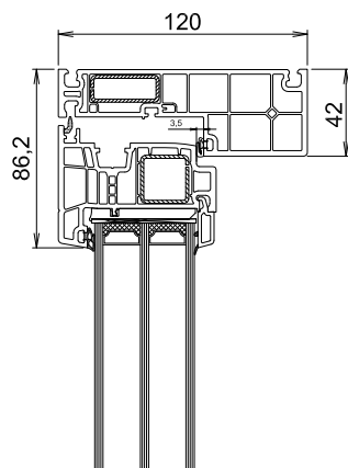
L20 = 76122(V312) - 76220(V556) - 76509
