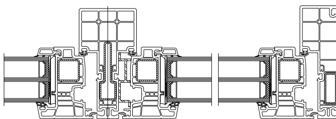
V21 = 76220(V556) - 76509 - 76318(V558)/A557 - 76220(V556)
