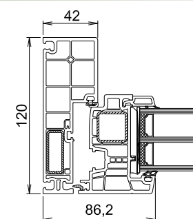
V20 = 76122(V312) - 76220(V556) - 76509
